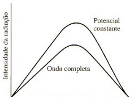
Figura 7 – Espectro dos Raios X e forma da onda aplicada
