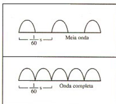
Figura 6 – Forma da onda aplicada em um tubo de Raios X
