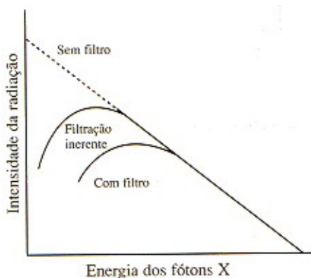
Figura 9 – Modificação do espectro dos Raios X pelo uso dos filtros
