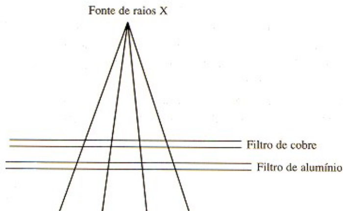
Figura 11 – Disposição dos filtros de cobre e alumínio
