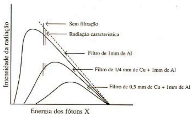
Figura 10 – Os filtros e os espectros dos Raios X
