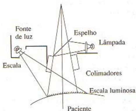
Figura 2 – Ilustração do campo luminoso
