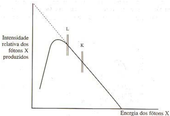
Figura 3 – Espectro total dos Raios X
