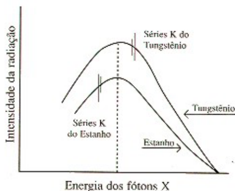
Figura 5 – Espectro dos Raios X e material do alvo
