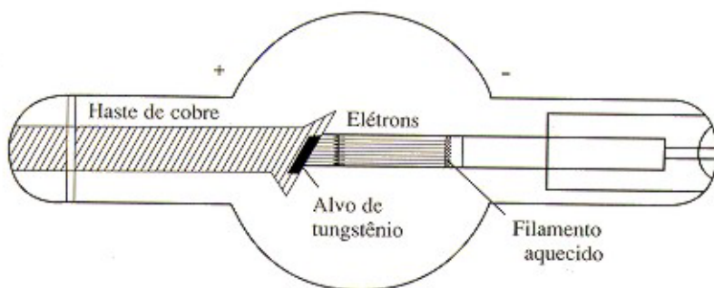
Figura 1 – Tubo de Raios X
