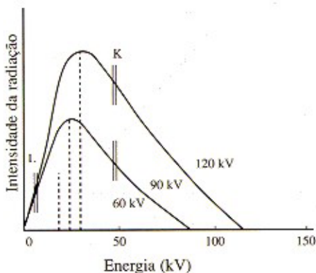
Figura 4 – Variação do espectro dos Raios X pela variação da kV
