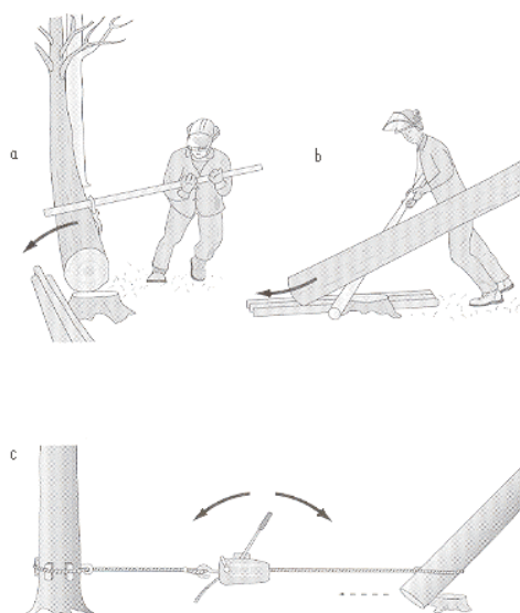
Figura 8 Práticas recomendadas para a derrubada de árvores enganchadas
