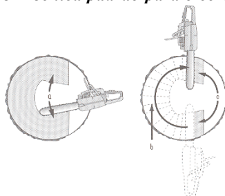
Figura 6b Técnica padrão para o corte de árvores
