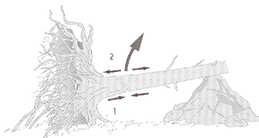
Figura 9b Traçamento de madeira sob tensão
