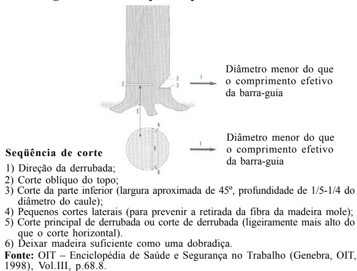
Figura 6a Técnica padrão para o corte de árvores
