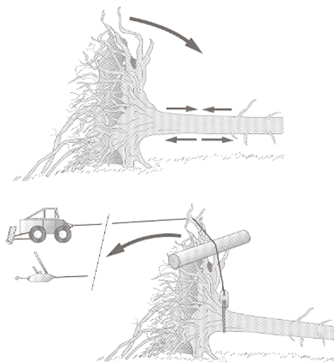
Figura 11 Separação das placas de raiz em árvores danificadas pelo vento
