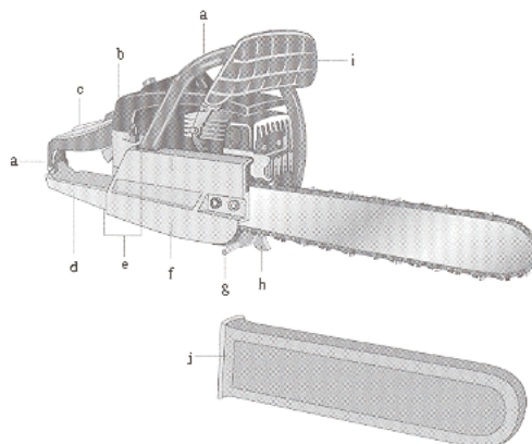
Figura 4 Dispositivos de segurança nas motosserras
